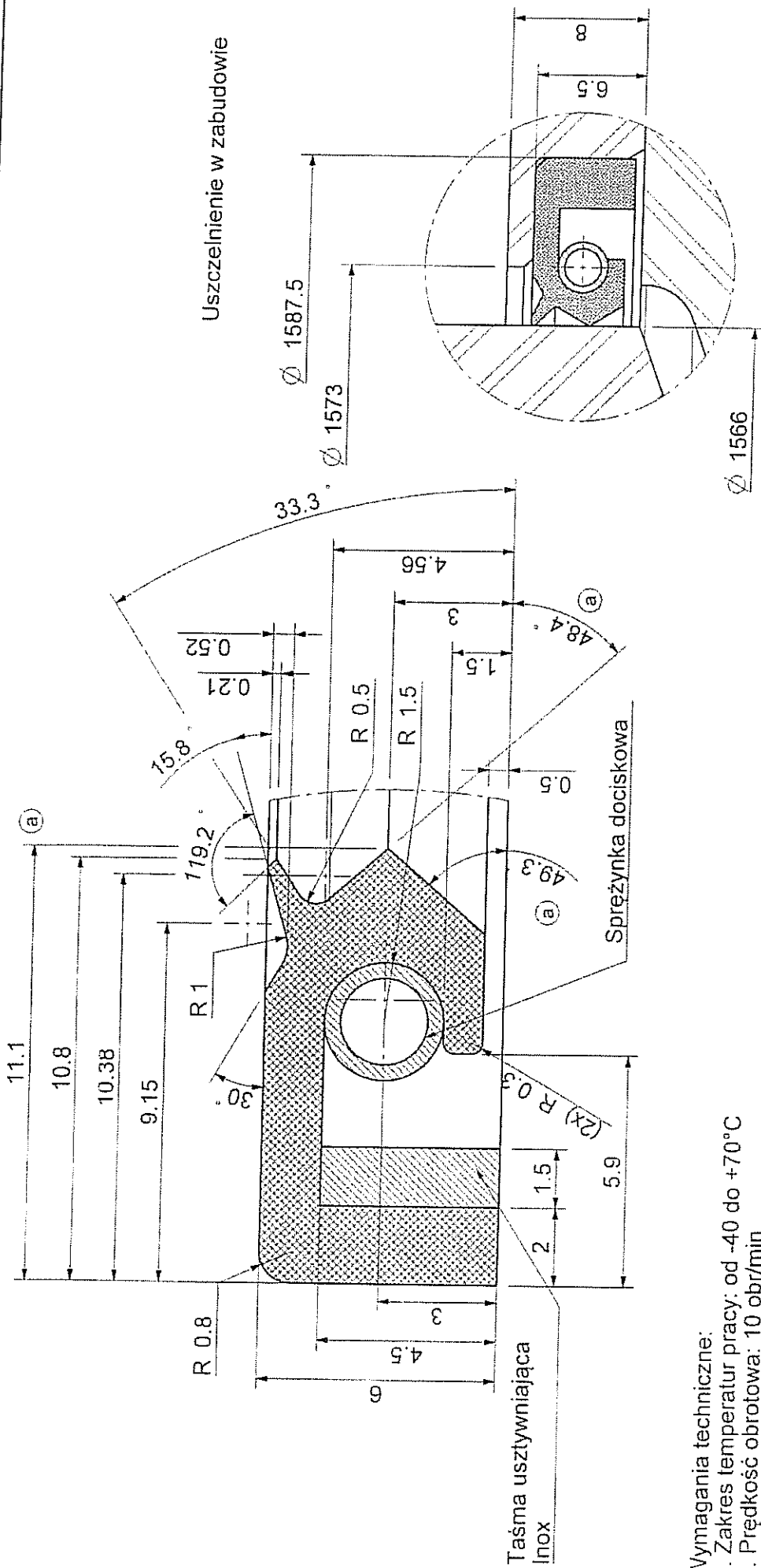
Rysunek do zapytania ofertowego
